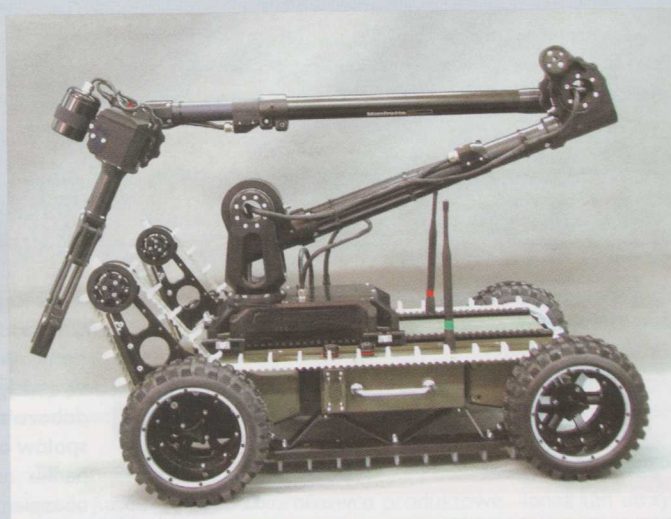
PIAP zrealizował kolejne dostawy robotów PIAP Gryf dla południowokoreańskich i indonezyjskich sił zbrojnych / Zdjęcie: PIAP
